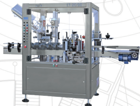
OMB / Z-Italia Etikettierer 1.000 Fl/h bis 50.000 Fl/h
